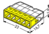
2273-205 5-conductor
